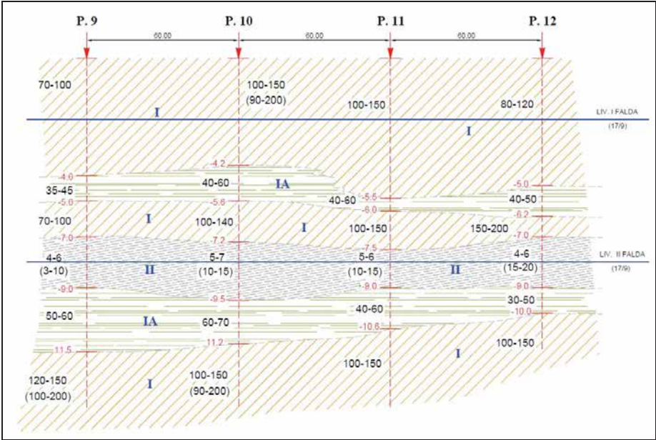
Figura 8: Sezione litostratigrafica P9-P10-P11-P12.
