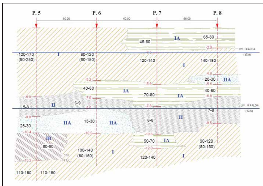
Figura 7: Sezione litostratigrafica P5-P6-P7-P8.
