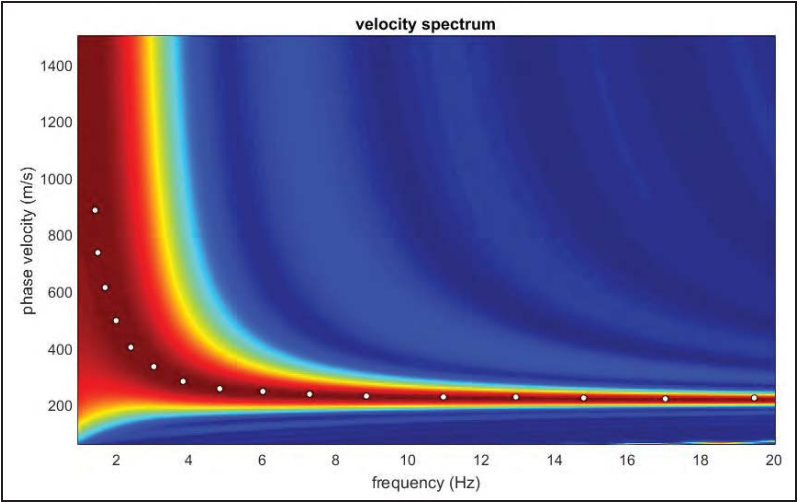
Figura 10: Spettro di velocità base sismica L1 con picking.
