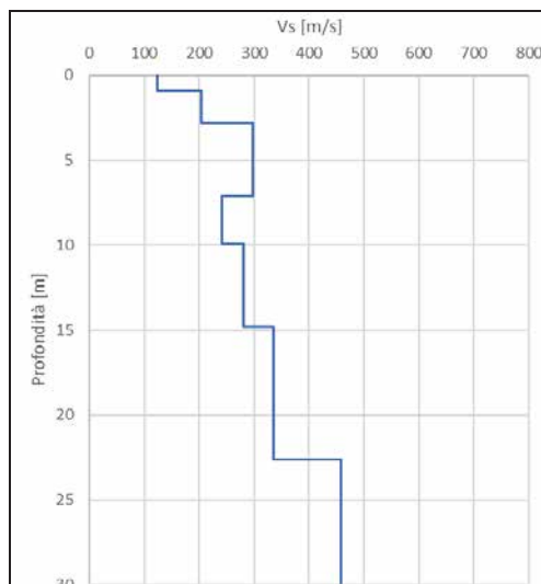
Figura 11: Diagramma delle velocità V_s riferite ai vari strati intercettati nella base sismica L1.
