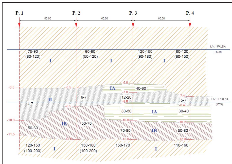
Figura 6: Sezione litostratigrafica P1-P2-P3-P4.
