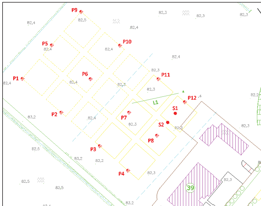
Figura 5: Planimetria con ubicazione indagini.
