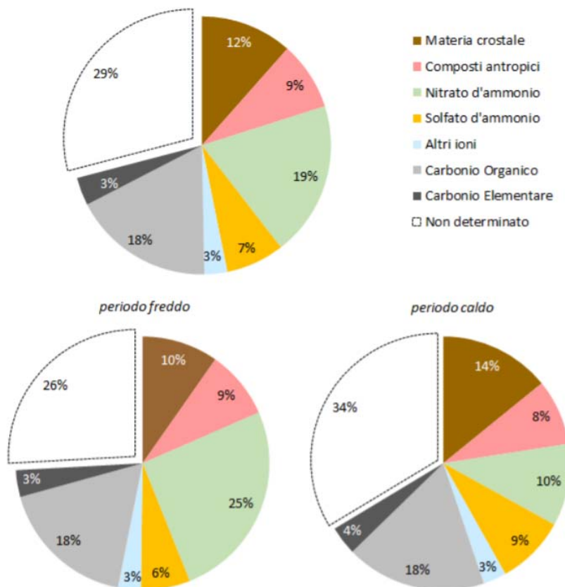
Composizione chimica del PM10 - MI-Marche
