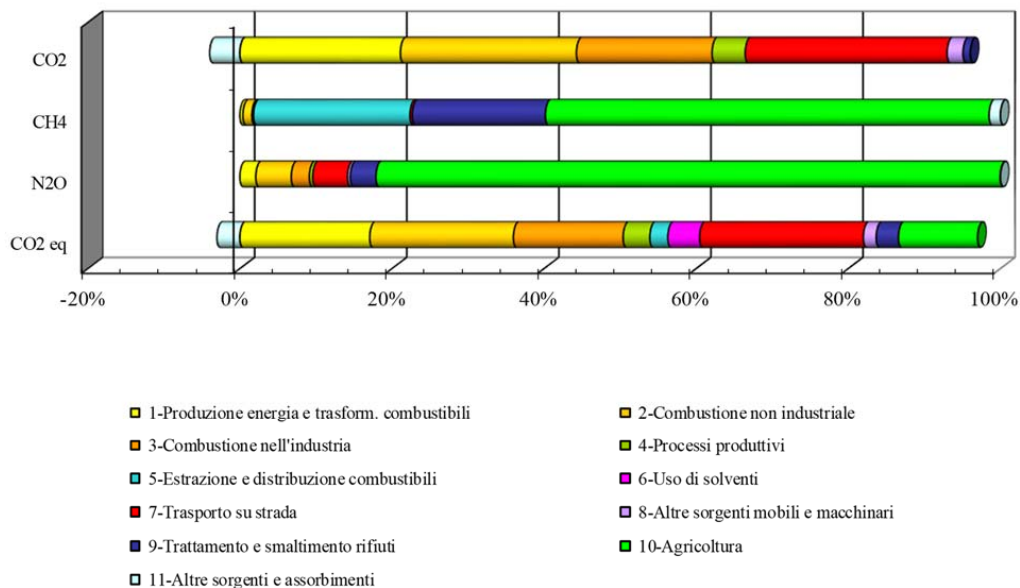
Figura 1.5. Emissioni di gas climalteranti nel 2017 in Lombardia suddivisi per inquinante e per macrosettore SNAP (Fonte: INEMAR ARPA LOMBARDIA).
