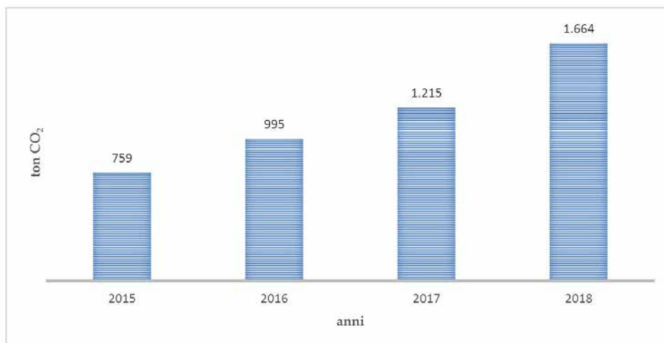
Fig. 1.29: Emissioni di CO 2 evitate (t) dai rispondenti al questionario (Elaborazione ENEA 2020)
