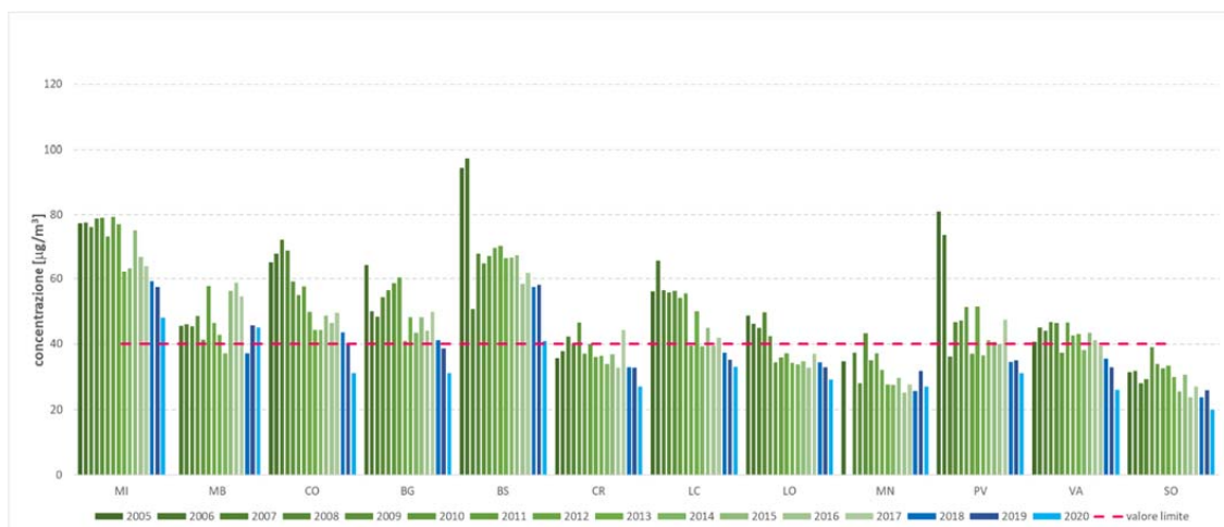
Fig. 4.10: Media annua di NO 2 nelle stazioni dei capoluoghi (stazione con valore massimo)
