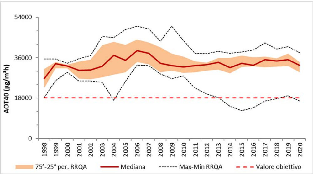
Fig. 4.27: trend AOT40 medio su 5 anni
