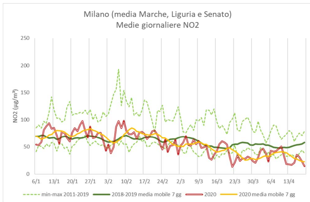
Fig. 1.20: dati di NO 2 del primo trimestre 2020 a confronto con quelli rilevati nel decennio a Milano
