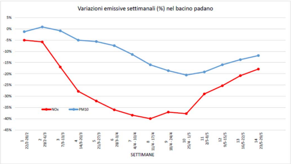
Figura 1.17 - Variazioni emissive settimanali (%) di NOx e PM10 nel bacino padano (22 febbraio - 29 maggio 2020)
