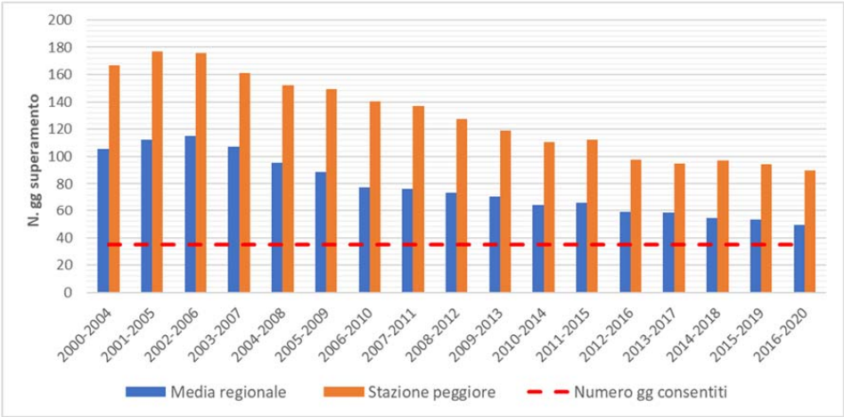
Fig. 4.4: Numero di giorni di superamento di PM10 raggruppati per quinquennio
