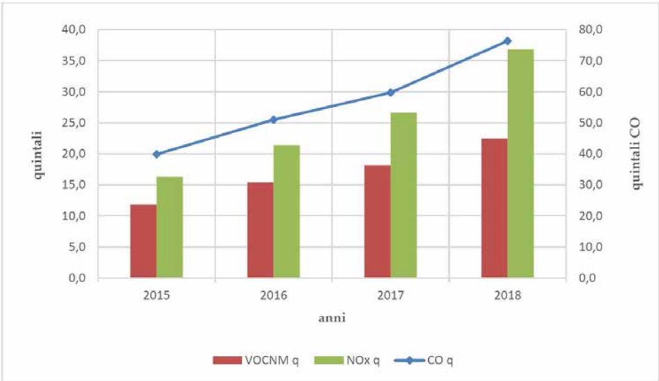
Fig. 1.30: Emissioni di composti organici volatili (non metanici), di ossidi di azoto e di monossido di carbonio evitate (q) dai rispondenti al questionario – Fonte studio ENEA citato
