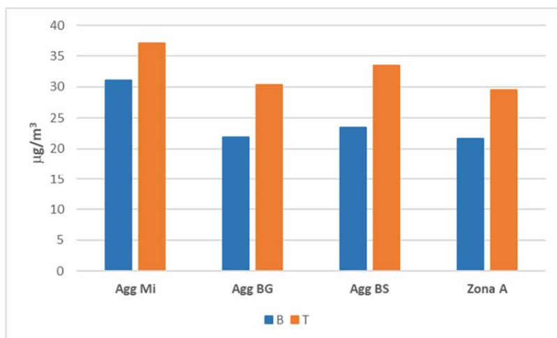
Fig 4.15: Media di NO2 nelle stazioni di background (B) e da traffico (T) anno 2020
