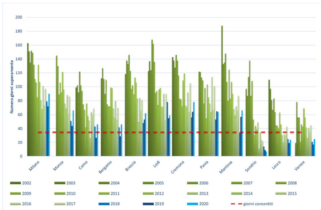
Fig. 4.2: Numero di giorni di superamento nelle stazioni dei capoluoghi
