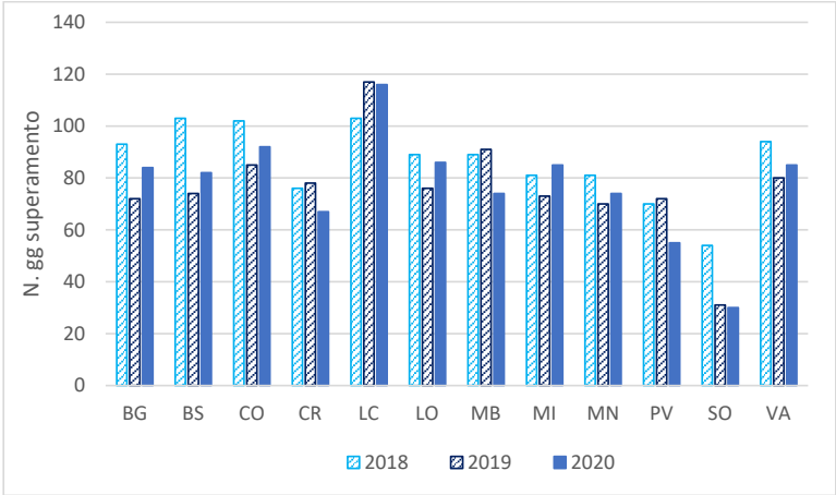
Fig. 4.16: Numero di giorni di superamento della massima media mobile per l’ozono nelle province
