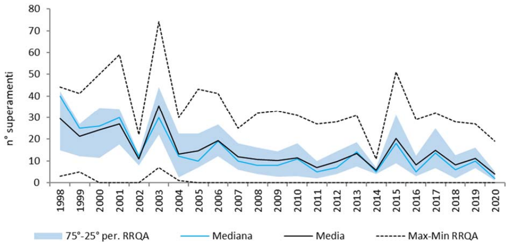
Fig 4.20: Andamento del n° di giorni di superamento della soglia di informazione (180 µg/m³)
