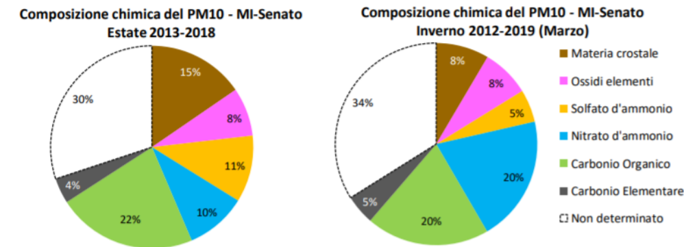
Fig.1.25 Elaborazione delle torte di chiusura di massa medie del PM10 di MI-Senato per i semestri estivo ed invernale.
