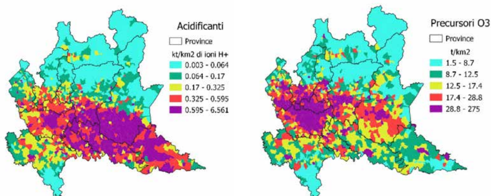
Figura 1.9. Mappa di emissione nel 2017 in Lombardia di Acidificanti e Precursori ozono (Fonte: INEMAR ARPA LOMBARDIA).
