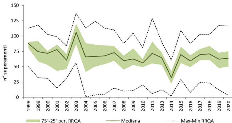
Fig 4.18: Andamento del numero di superamenti annuali dell'obiettivo a lungo termine per l'O3
