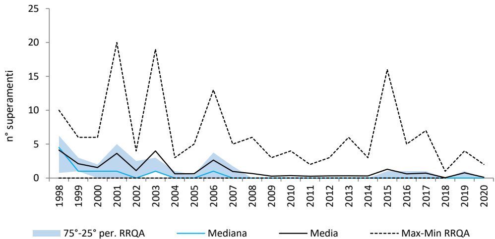
Fig 4.21: Andamento del n° di giorni di superamento della soglia di allarme (240 µg/m³)
