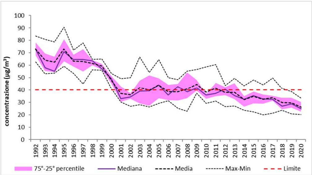
Fig 4.13: Andamento delle concentrazioni medie annuali di NO2 nell’Agglomerato di Bergamo
