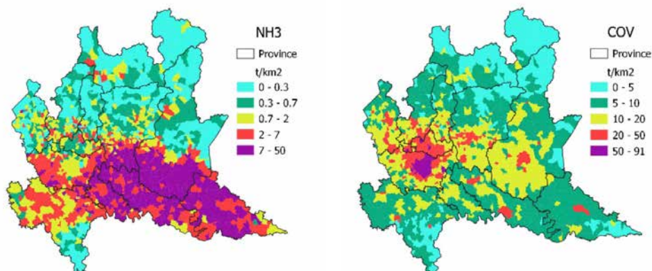
Figura 1.7. Mappe di emissione nel 2017 in Lombardia per \text{PM}_{10} , \text{NO}_x , \text{NH}_3 e COVNM (Fonte: INEMAR ARPA LOMBARDIA).
