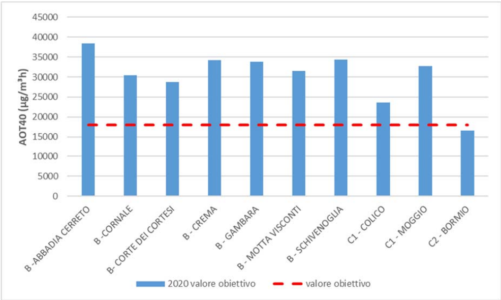
Fig. 4.25: AOT40 medio su 5 anni nel 2020
