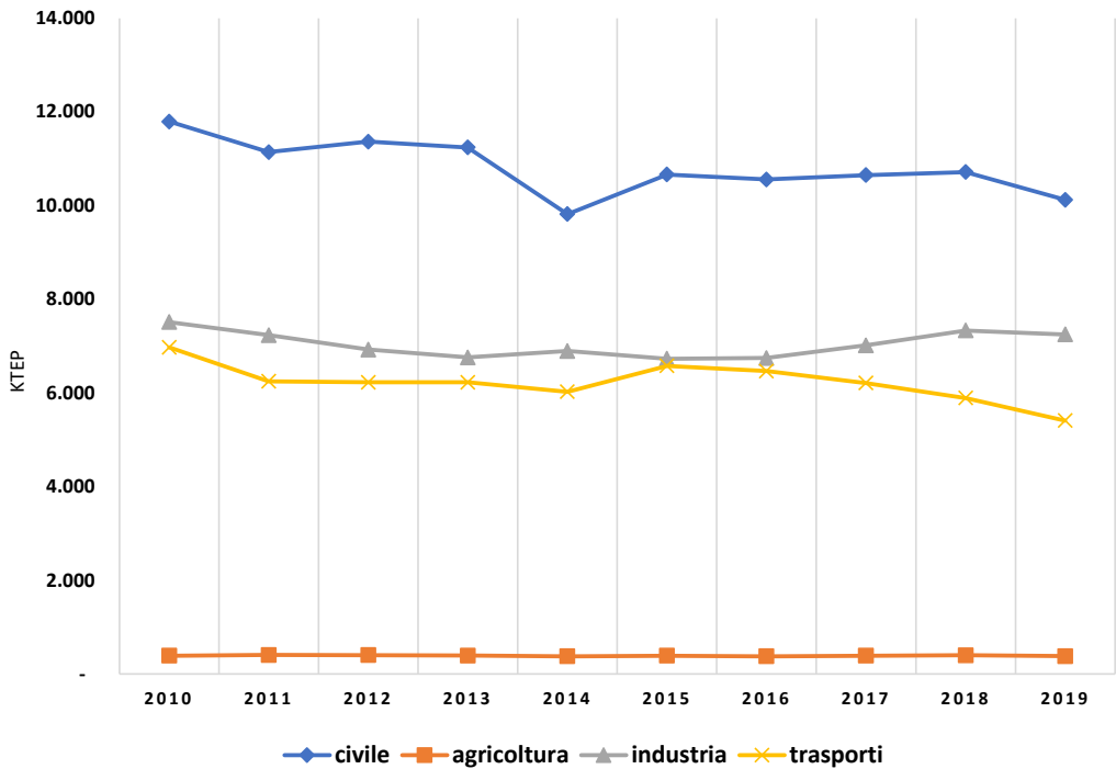
Fig. X – Andamento dei consumi di energia finale per settore in Lombardia (2010-2019). Fonte: Elaborazioni ARIA S.p.A., Sistema Informativo Regionale Energia e Ambiente.
