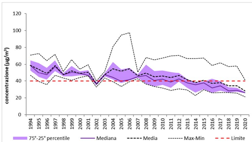
Fig 4.14: Andamento delle concentrazioni medie annuali di NO2 nell'Agglomerato di Brescia
