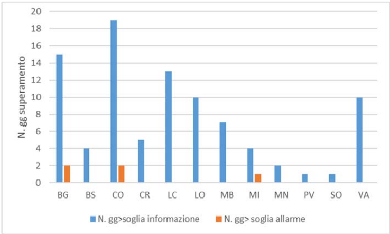
Fig. 4.17: Numero di giorni per provincia in cui si è registrata almeno un’ora di superamento della soglia di informazione e di allarme per l’ozono nel 2020
