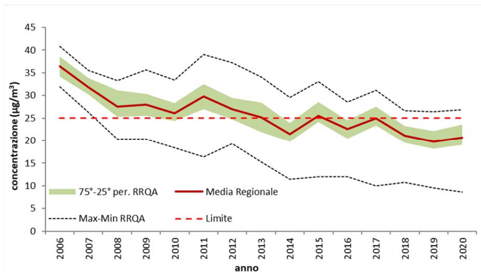
Fig. 4.9: Andamento delle concentrazioni medie annuali di PM2.5 Regione Lombardia
