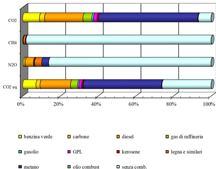
Figura 1.6. Emissioni di gas climalteranti nel 2017 in Lombardia suddivisi per inquinante e tipologia di combustibile (Fonte: INEMAR ARPA LOMBARDIA).
