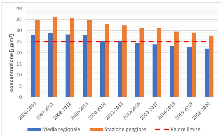
Fig. 4.8: Medie annue di PM2.5 raggruppate per quinquennio
