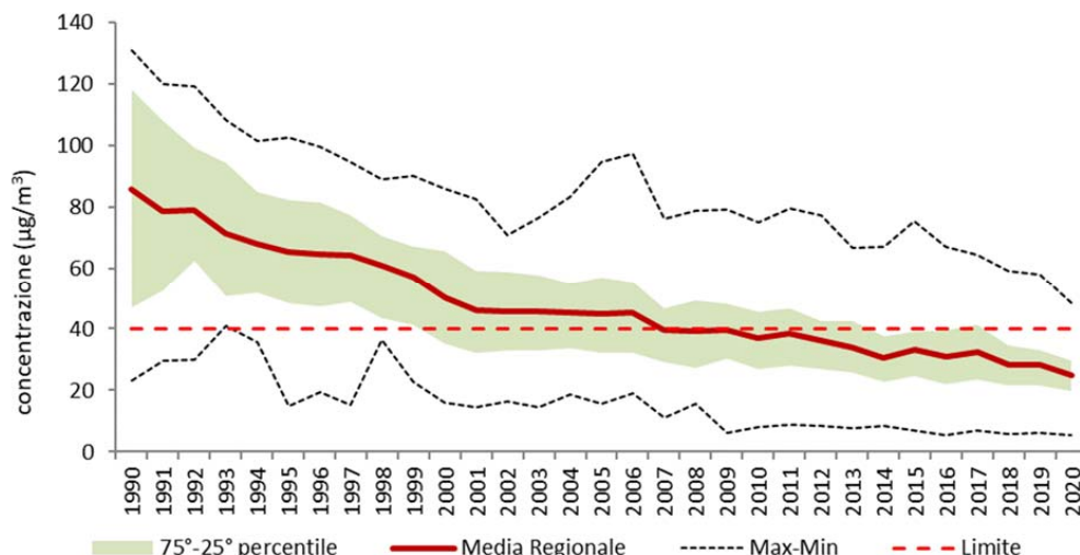
Fig 4.11: Andamento delle concentrazioni medie annuali di NO2 Regione Lombardia
