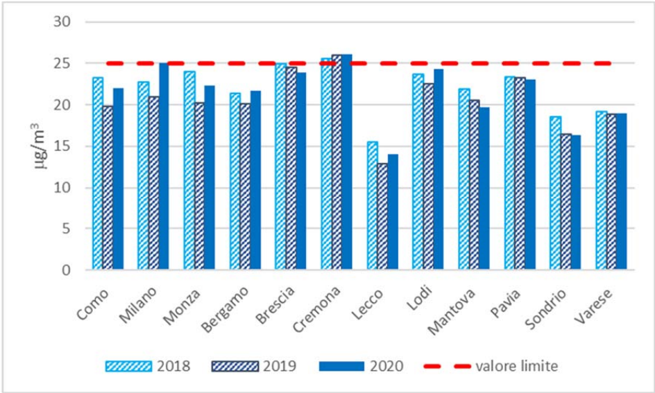
Fig. 4.7: Media annua di PM 2.5 nelle stazioni dei capoluoghi
