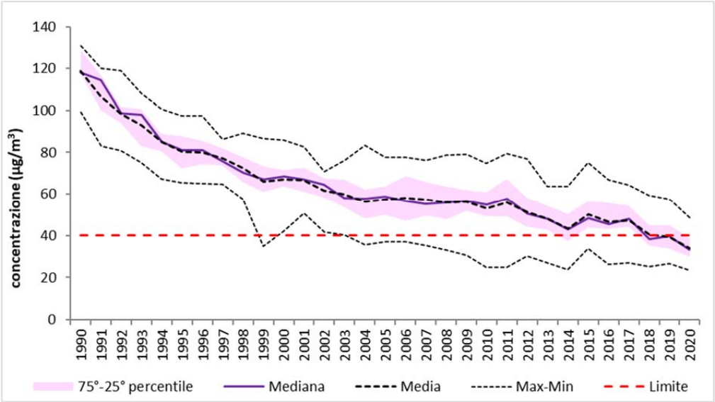
Fig 4.12: Andamento delle concentrazioni medie annuali di NO2 nell’Agglomerato di Milano
