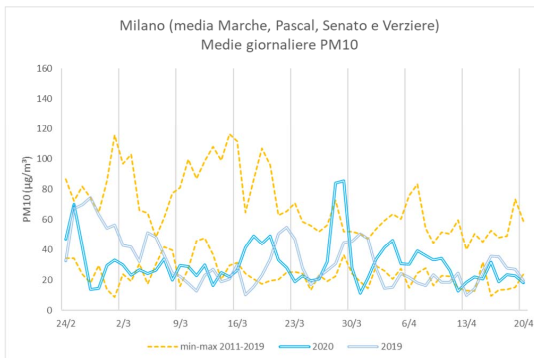
Fig. 1.21: dati di PM10 fra fine febbraio e aprile 2020 a confronto con quelli rilevati nel decennio a Milano
