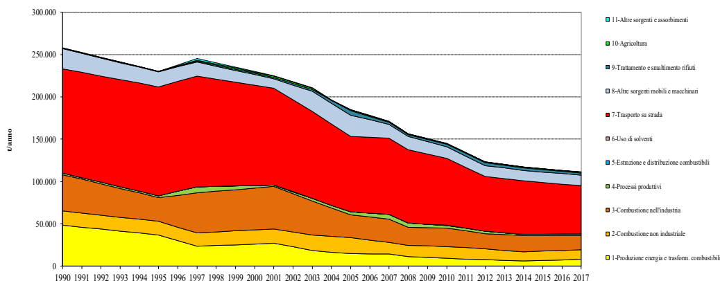
Figura 1.4. Serie storica delle emissioni di NO x (t/anno) in Lombardia. Fonte: elaborazioni ARPA Lombardia
