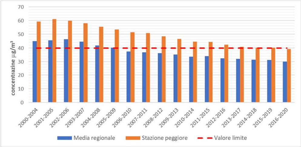
Fig. 4.3: Medie annue di PM10 raggruppate per quinquennio
