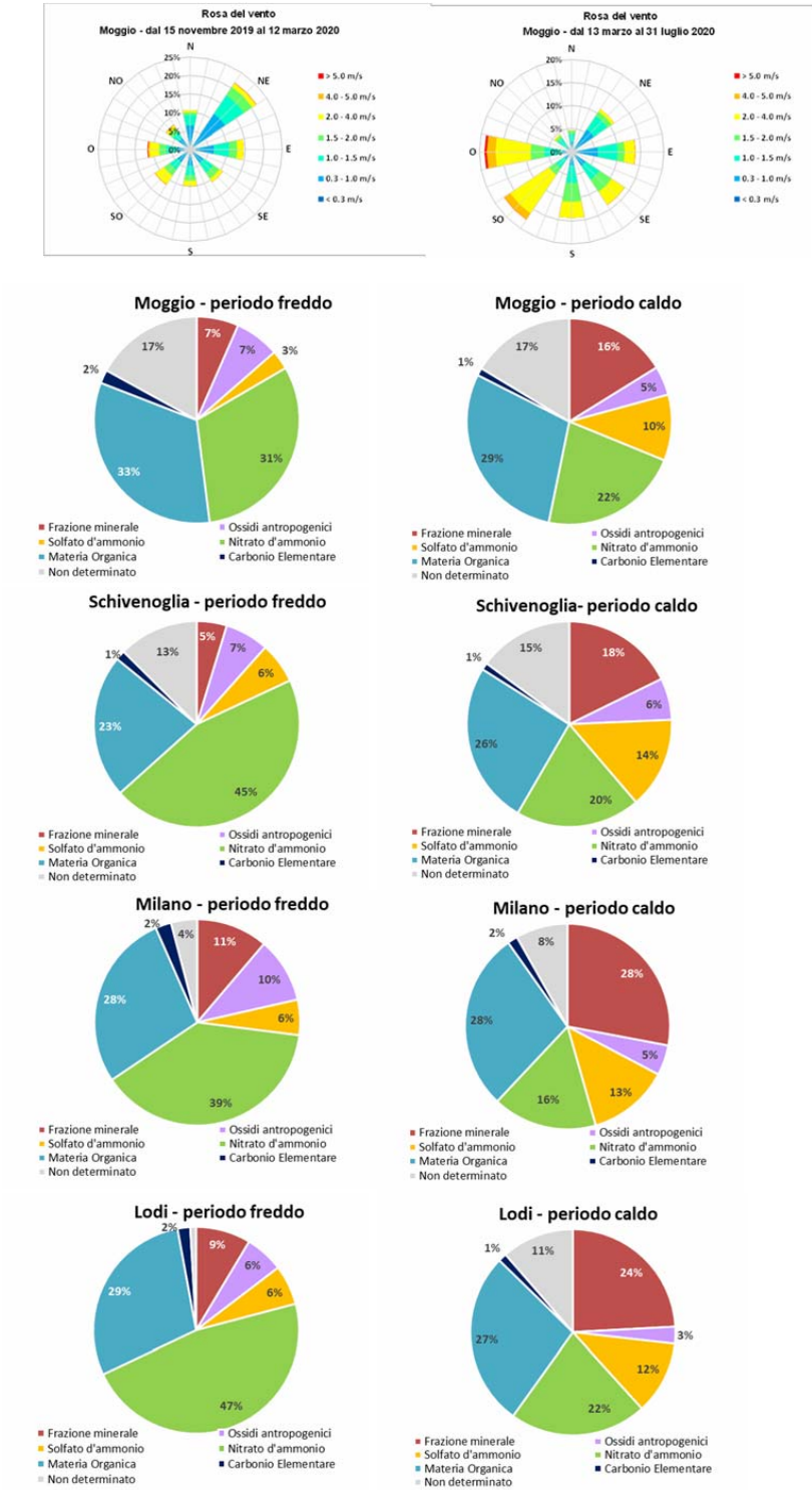
Figura 1.28: Composizione chimica del PM10 misurato a Moggio, Milano, Lodi, Schivenoglia nel periodo freddo (dal 15 novembre 2019 al 12 marzo 2020) e caldo (dal 13 marzo a 1°agosto 2020) della campagna.
