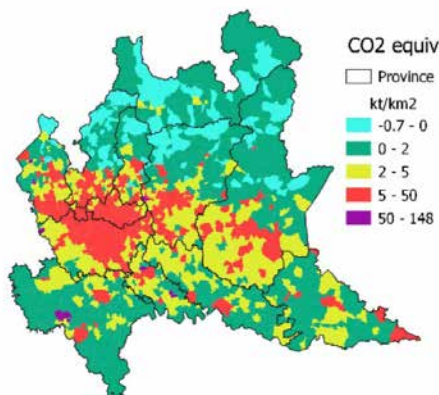
Figura 1.8. Mappa di emissione nel 2017 in Lombardia di \text{CO}_2 equivalente (Fonte: INEMAR ARPA LOMBARDIA).
