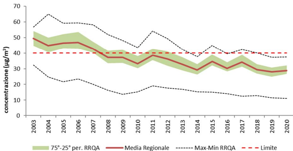
Fig. 4.5: Andamento delle concentrazioni medie annuali di PM10 Regione Lombardia
