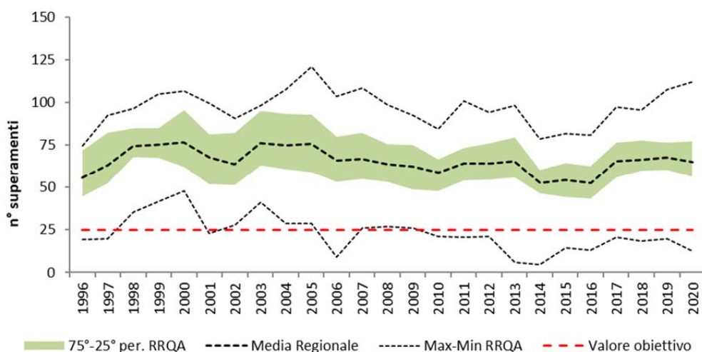
Fig 4.19: Andamento del numero di superamenti annuali dell'obiettivo a lungo termine per l'O3 (media su 3 anni)
