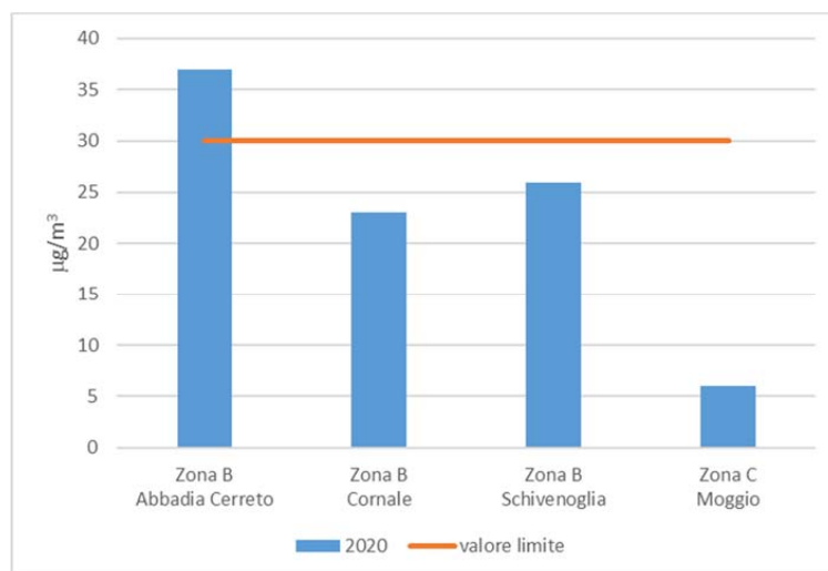
Fig. 4.23: Media annuale di NOX 2020
