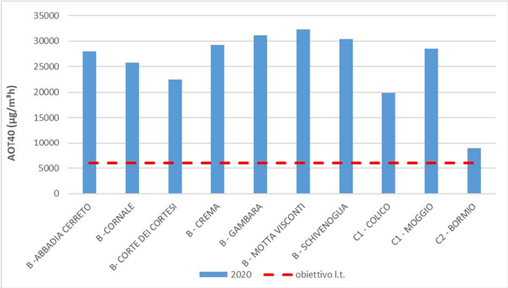
Fig. 4.24: AOT40 annuale nel 2020
