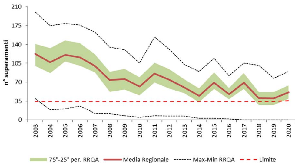
Fig. 4.6: Andamento del n° di superamenti annuali di PM10 Regione Lombardia
