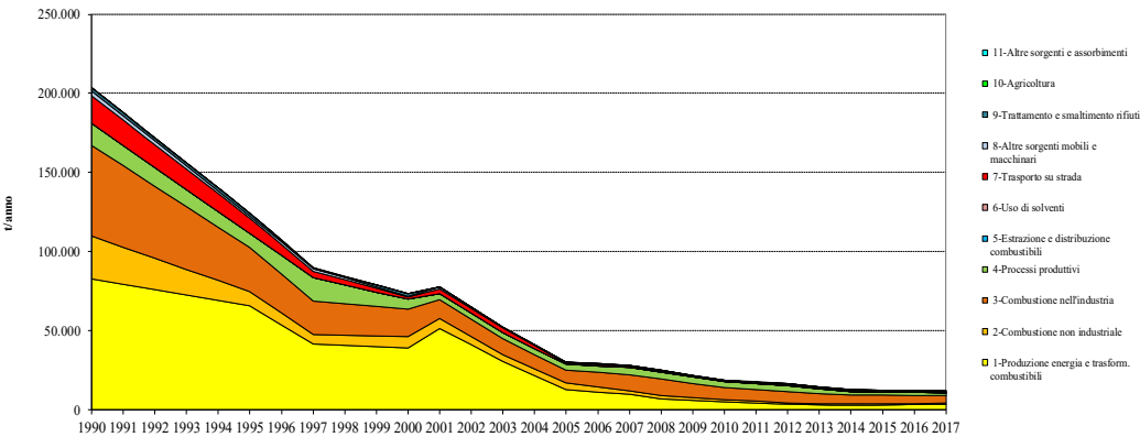
Figura 1.3. Serie storica delle emissioni di SO 2 (t/anno) in Lombardia. Fonte: elaborazioni ARPA Lombardia.
