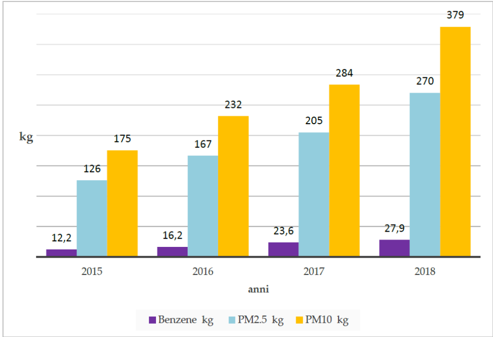
Fig. 1.31: Emissioni di benzene, di PM 2,5 e di PM10 evitate (kg) dai rispondenti al questionario – Fonte studio ENEA citato
