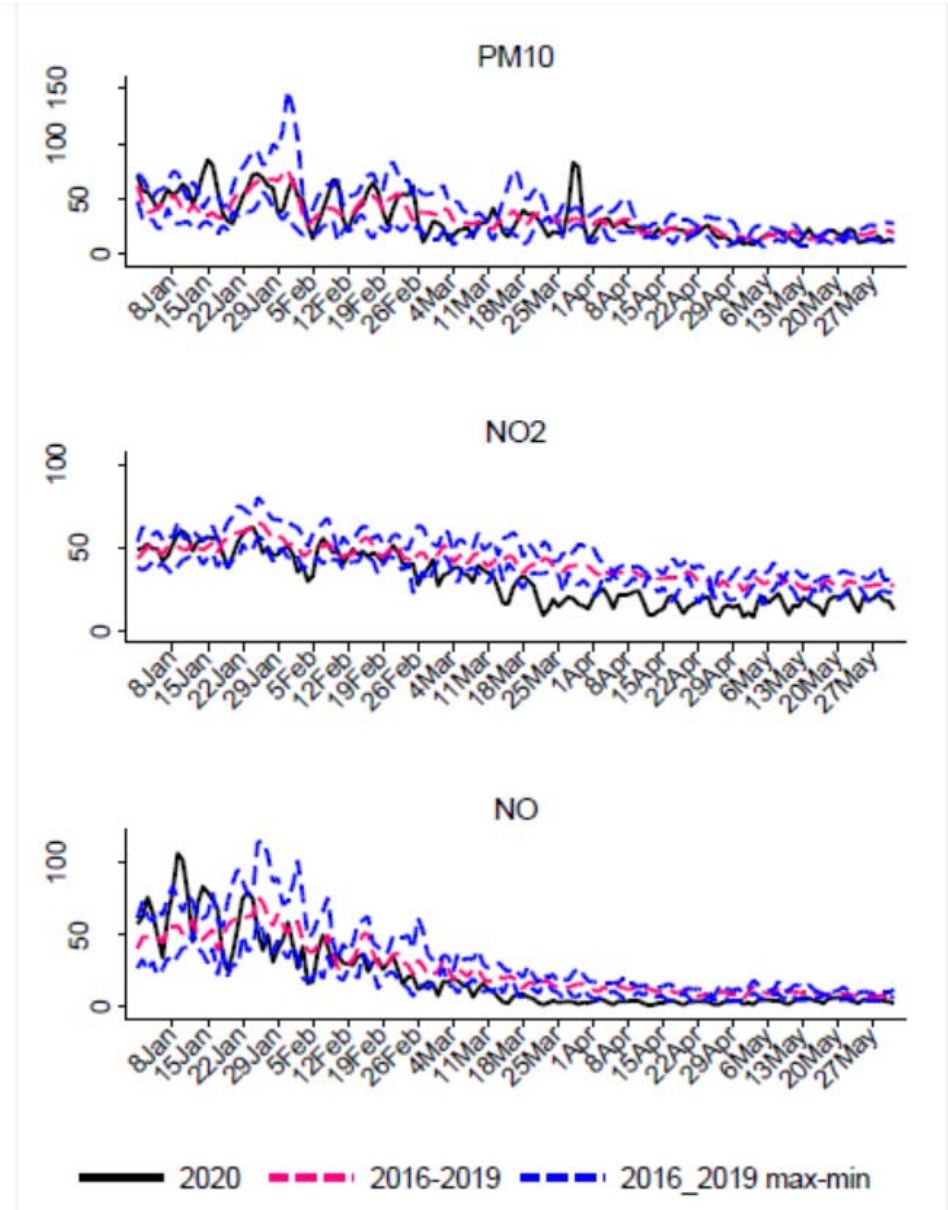
Figura 1.18 – Confronto tra l’andamento giornaliero delle concentrazioni medie di PM10, NO2 e NO (media di tutte le stazioni da traffico) dei mesi di gennaio, febbraio, marzo, aprile e maggio 2020 e quello della media, della massima e
