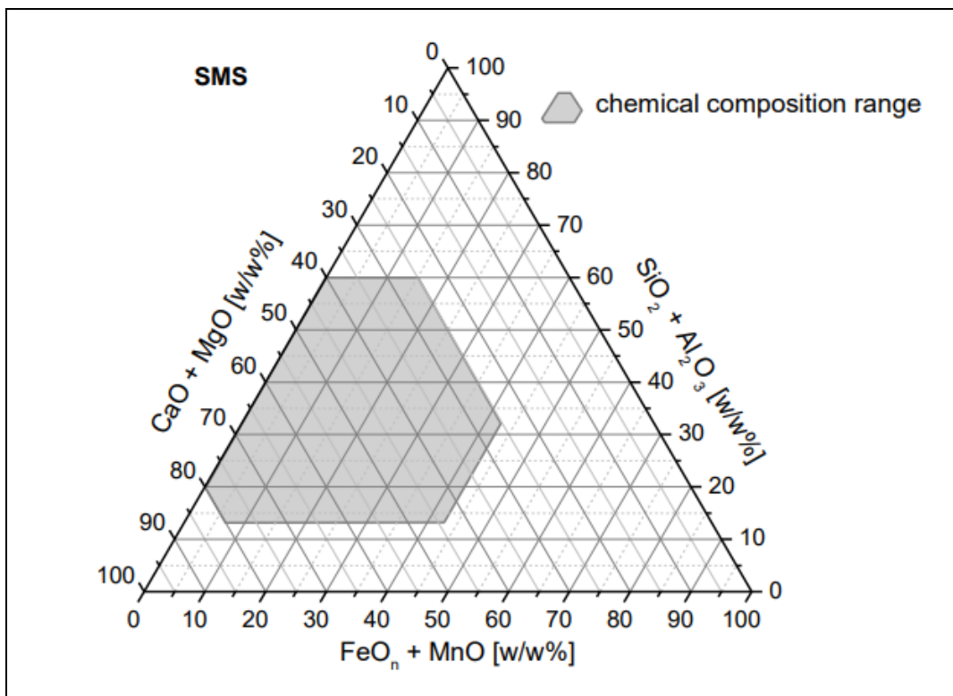
FIGURA 2 - DIAGRAMMA TERNARIO DELLA SCORIA BIANCA DA METALLURGIA SECONDARIA SMS.
