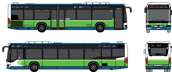
Per autobus extraurbani (esempio: bus a 2 porte)
